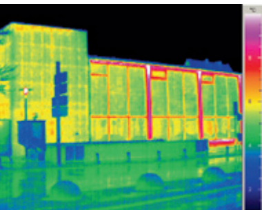
Wärmebild Markthalle Hannover
